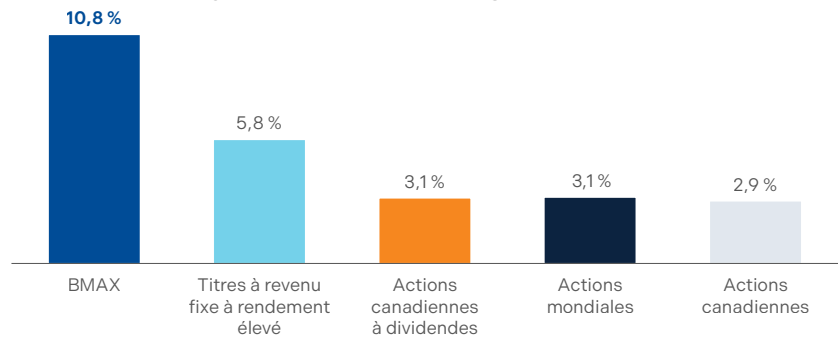
Distribution cible de BMAX par rapport à la distribution moyenne de chaque catégorie de fonds 5
